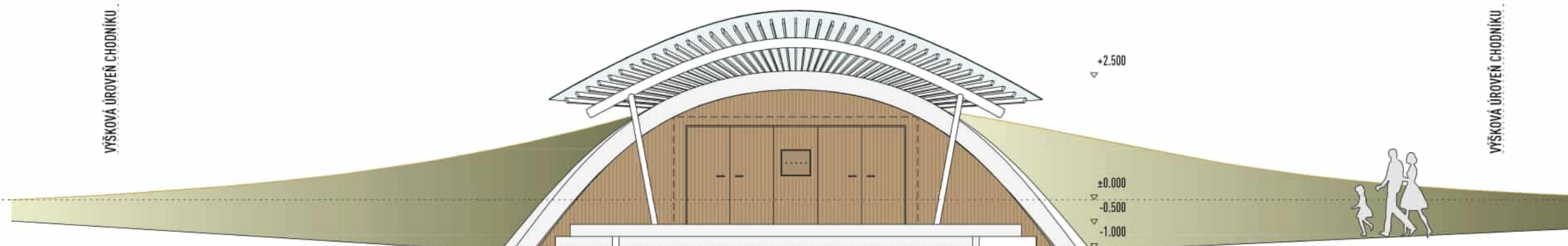
AMFITEÁTR - ČELNÍ POHLED
